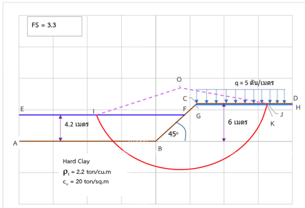
ภาพแสดงตัวอย่างการวิเคราะห์ค่าความมั่นคงของดิน (Soil Stability)
